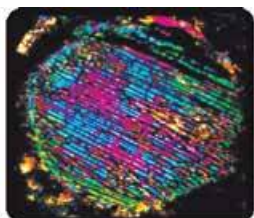
▲ مقطع میکروسکوپی از یک کندرول به اندازه یک میلی متر در یک شهاب سنگ کندریتی ۲ ، کانی ها به صورت تیغه های کشیده و موازی در کنار یکدیگر متبلور شده اند.
