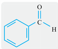
فرمول ساختاری و مدل فضای بنزآلدهید
